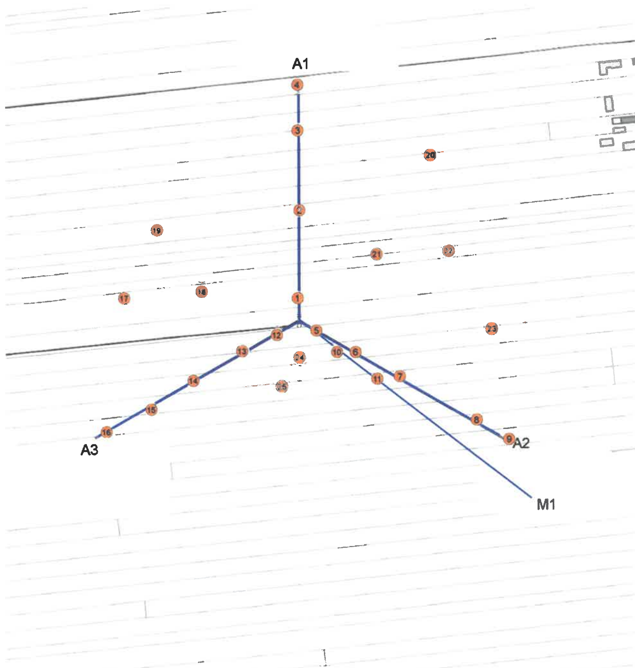
Azymuty anten
